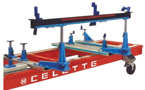
Portique de contrôle des côtés de caisse Checking overhead gantry for the upper panels of the car-body
