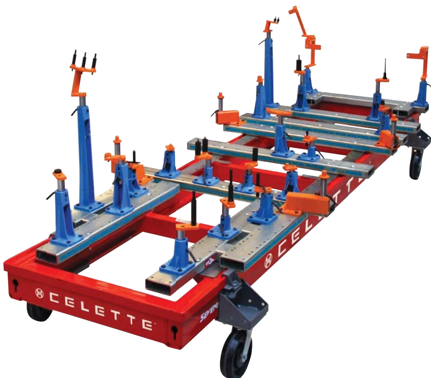
Le contrôle peut s'effectuer sur tous les marbres CELETTE mécanique en place ou mécanique déposée. Checking may be completed on all CELETTE benches, with or without mechanical units
